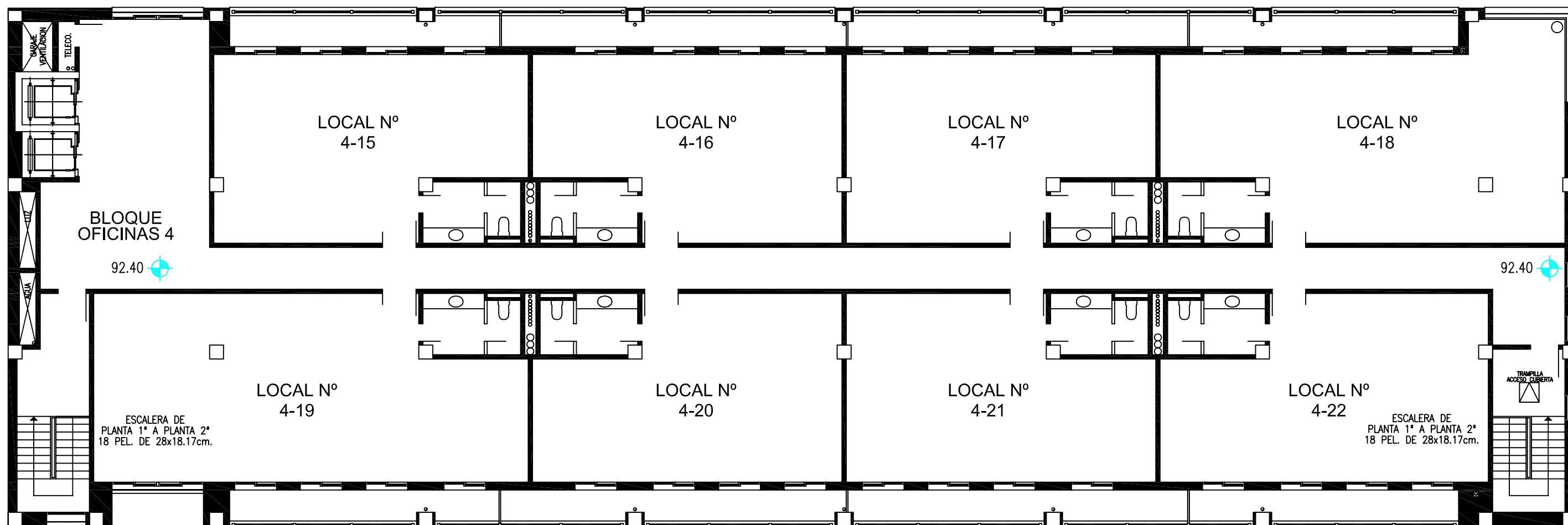
PLANTA 2ª. (BLOQUE 4).
