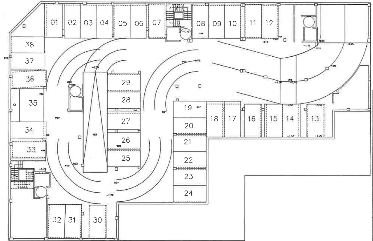
PLANTA SOTANO 1
