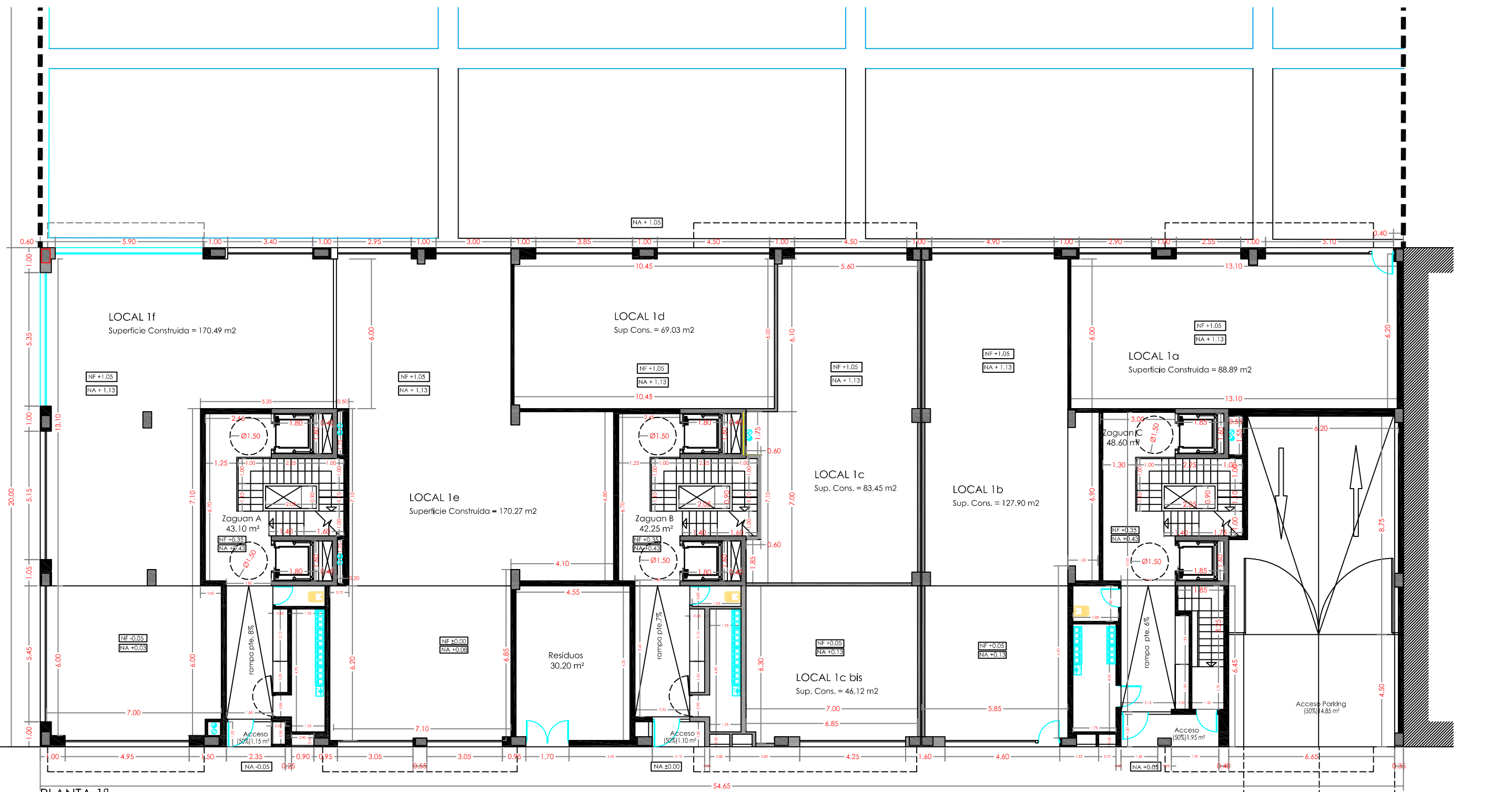
PLANTA 1ª
