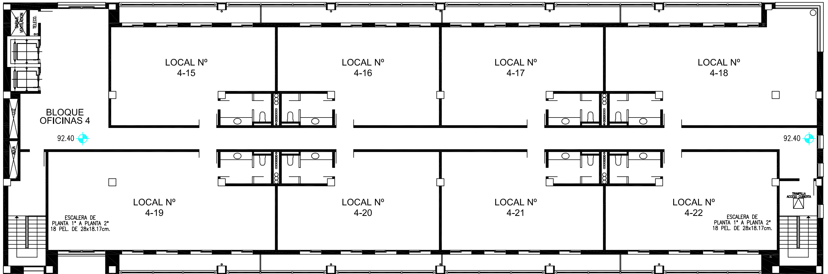
PLANTA 2ª. (BLOQUE 4).
